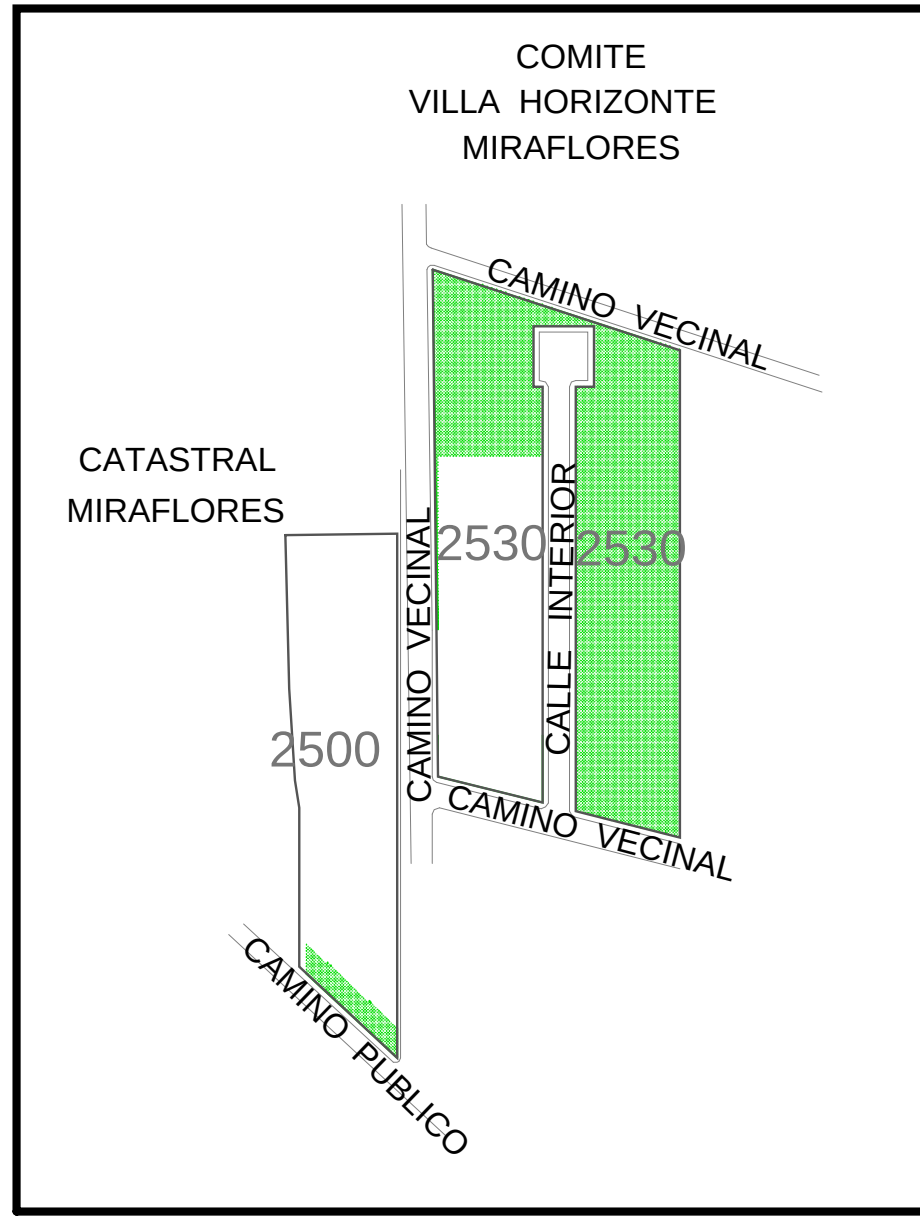
DETALLE ESCALA 1/2500
