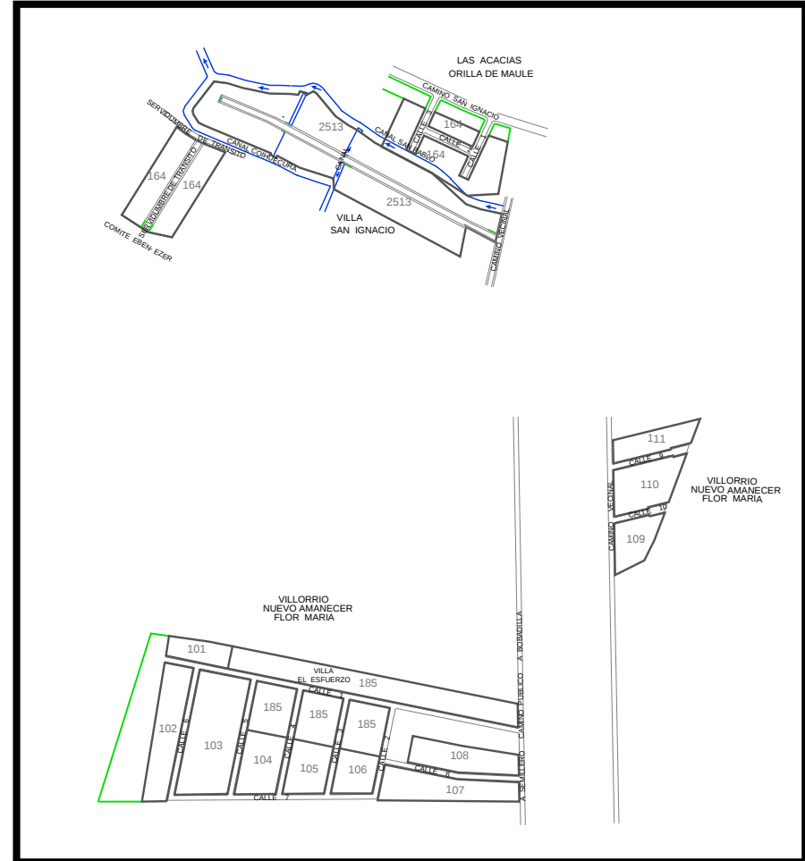
DETALLE ESCALA 1/10000
